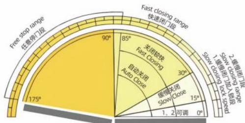
各门类定位功能示意图
