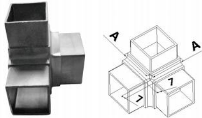
Item NO A T-33-4040 40X40 T-33-5050 50X50
