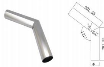
Item NO Ø T-32-508 50.8
