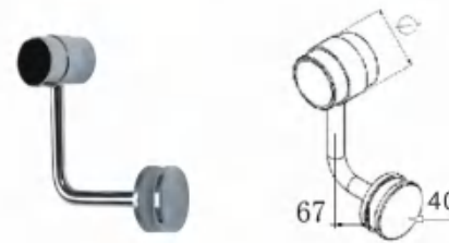
TJ-84 Item NO \phi TJ-84-508 50.8
