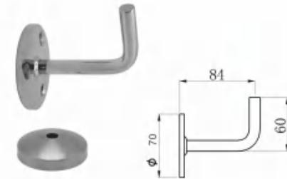
TJ-83 Item NO \phi TJ-83-70 70
