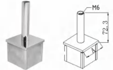
TJ-81 Item NO A TJ-81-4040 40×40 TJ-81-5050 50×50
